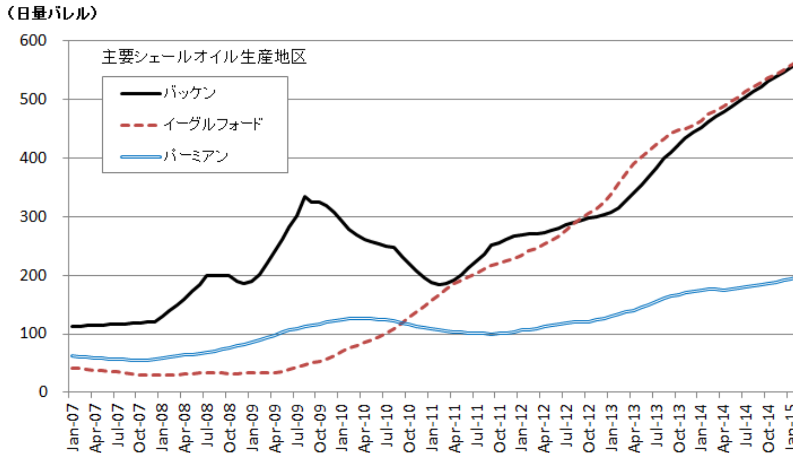
【図2】 新規1稼動リグ当たりの原油生産量
