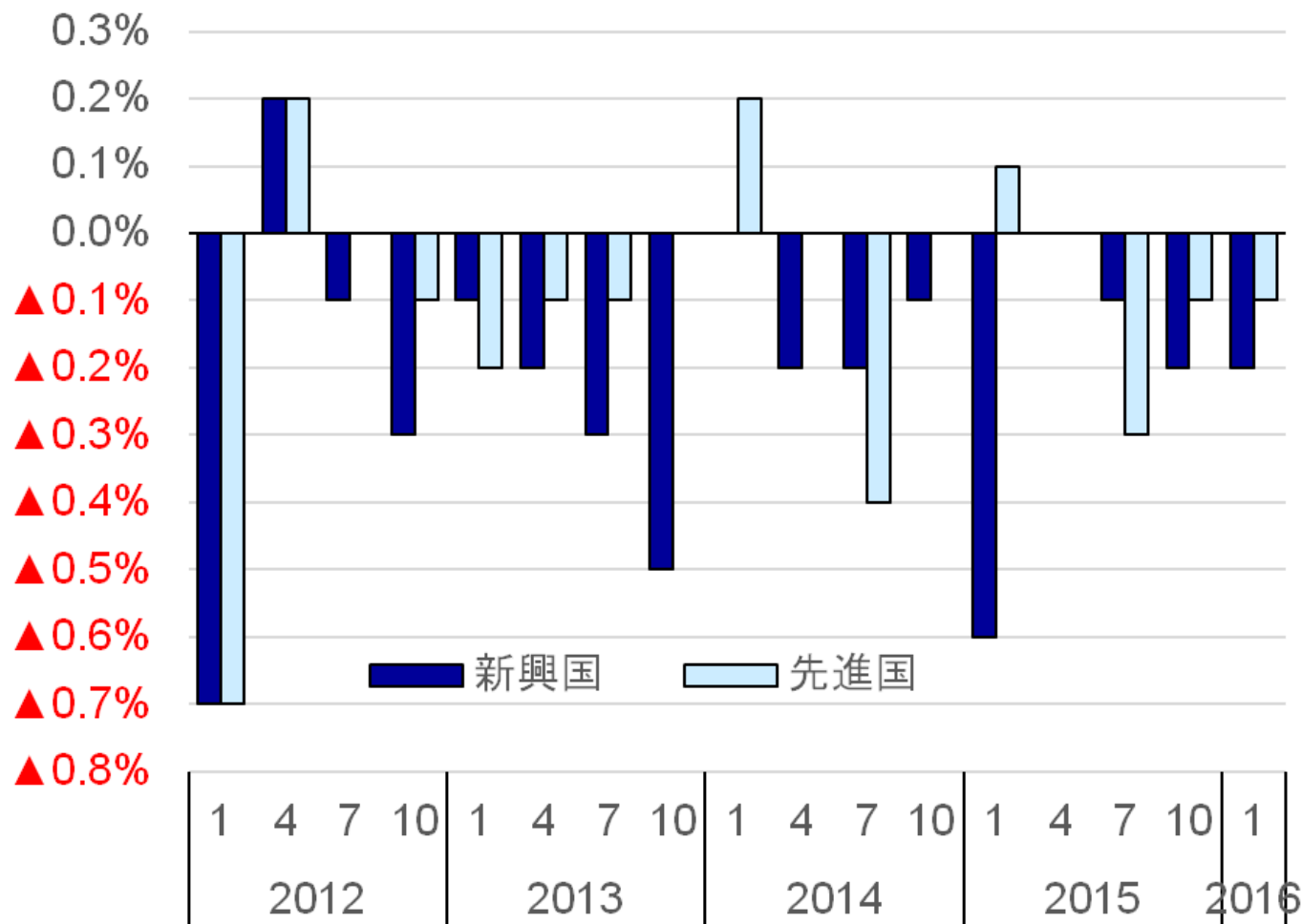
【図表1】 直近年の成長予測(IMF)の修正幅
