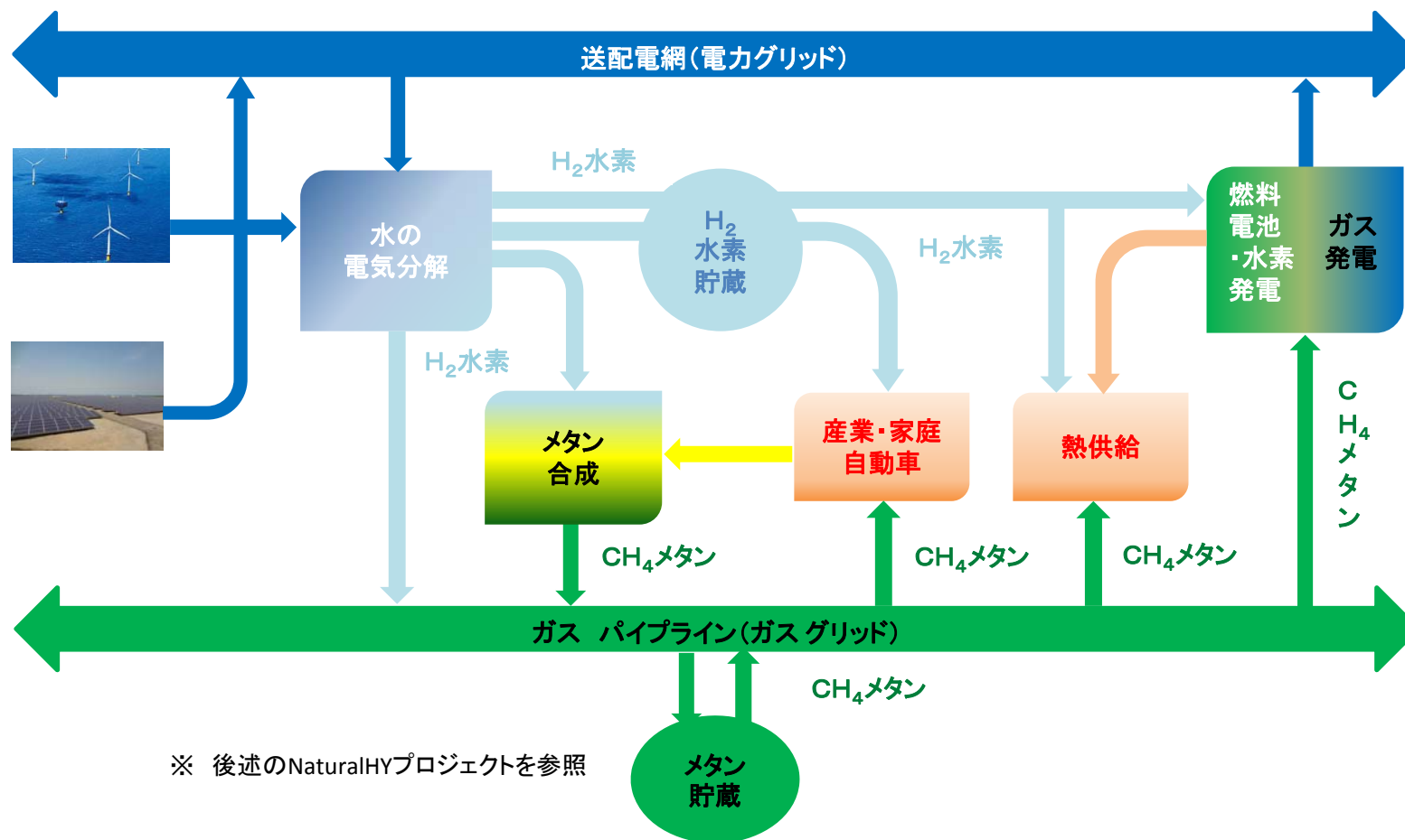
【図表 1】 Power-to-Gasのコンセプト
